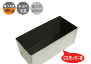
香蕉吐司盒 Banana Loaf Pan QN2150 表面处理: 砂利康不沾 上径尺寸 267x132x108.5mm 下径尺寸 267x119mm
