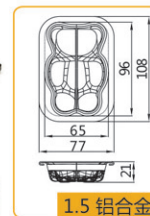
1.5 铝合金
